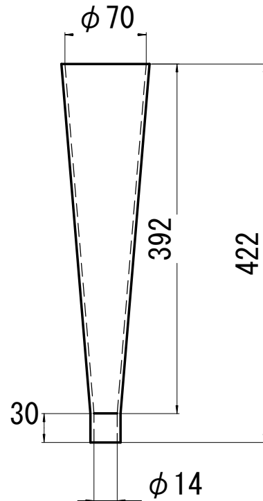
約630ml J P ロート (土木学会規準)
