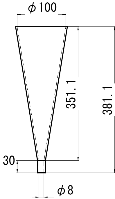
約1000ml J A ロート (土木学会規準)
