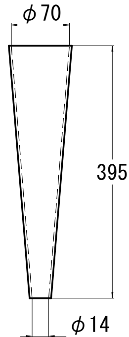
約630ml J ロート14 (道路公団規格)
